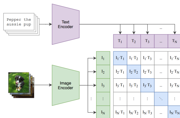
Рис. 76: Схема обучения CLIP. Взято из статьи “Learning Transferable Visual Models From Natural Language Supervision”.
