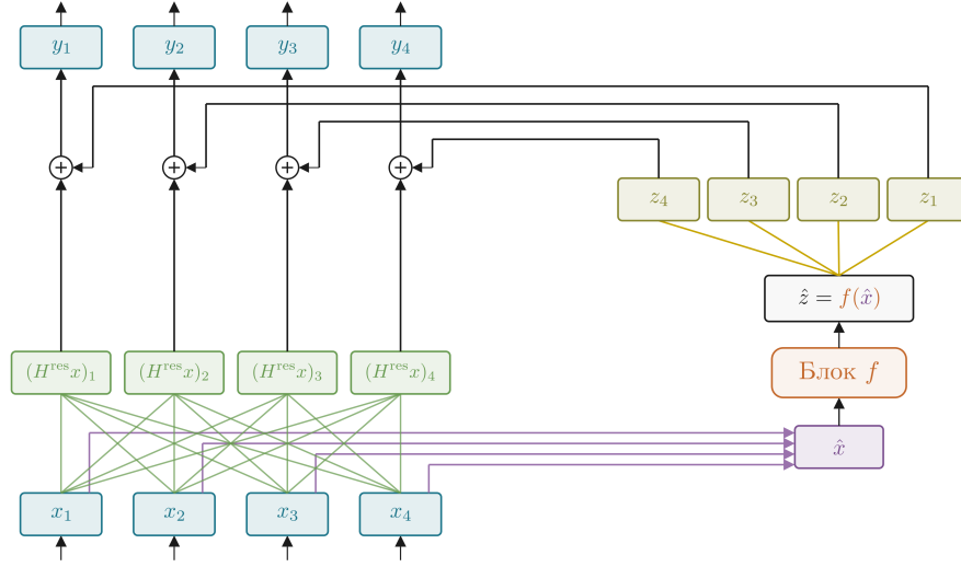
Рис. 66: Схема гиперсвязей одного слоя f трансформера.
