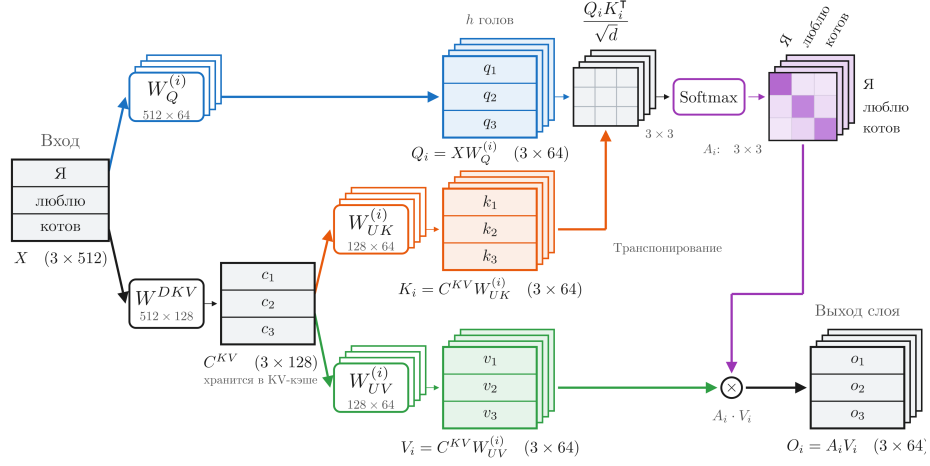
Рис. 70: Схема Multihead Latent Attention.
