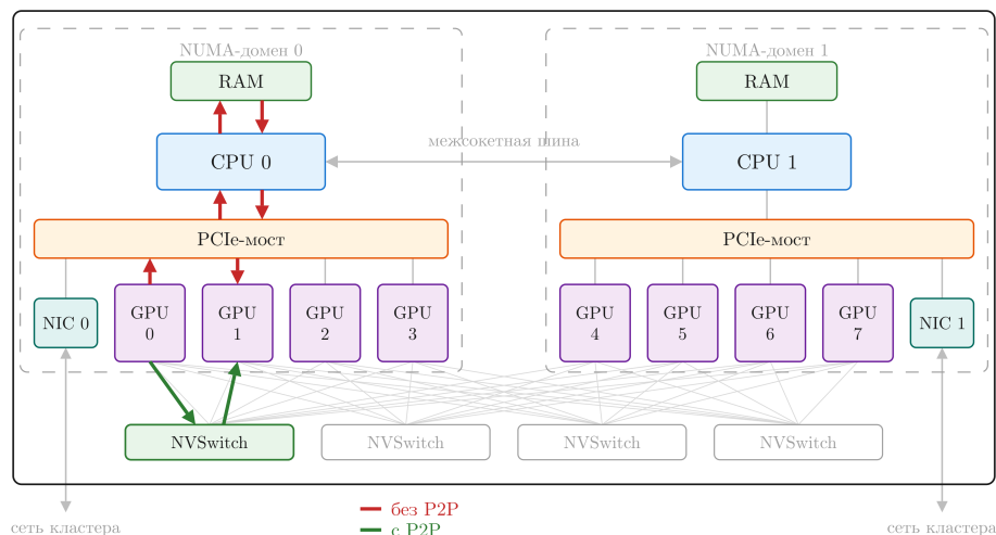
Рис. 34: Схема P2P-связи между GPU.
