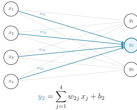
Рис. 1: Схема полносвязного слоя.
