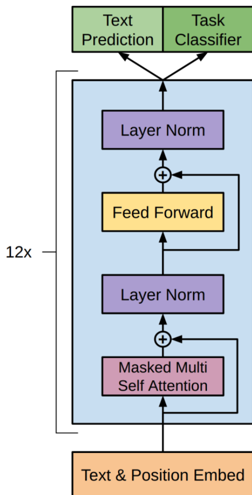
Рис. 75: Схема GPT-1. Взято из статьи “Improving Language Understanding by Generative Pre-Training”.
