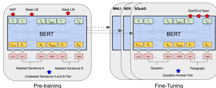
Рис. 74: Схема BERT. Взято из статьи “BERT: Pre-training of Deep Bidirectional Transformers for Language Understanding”.
