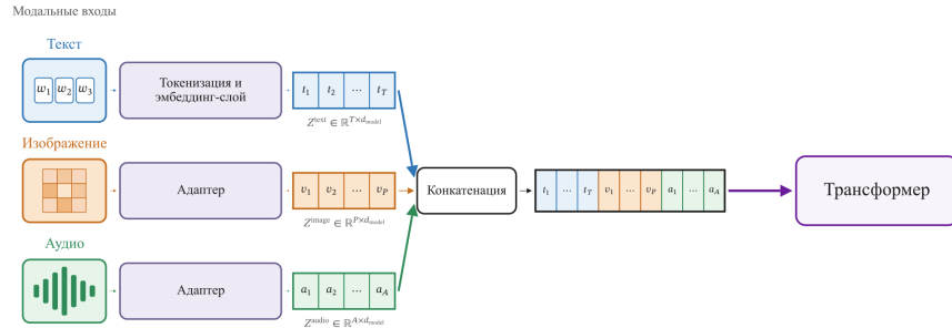
Рис. 77: Схема раннего смешивания модальностей.
