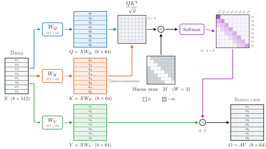
Рис. 72: Схема скольльзящего оконного внимания.
