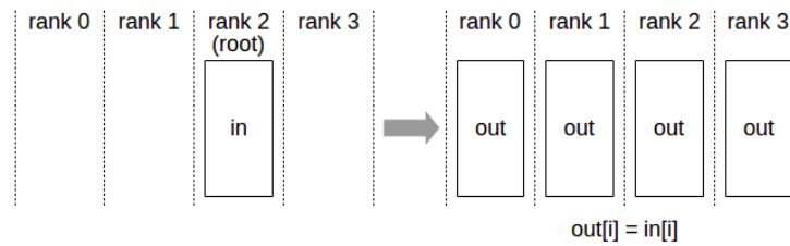
Рис. 38: Схема Broadcast.
