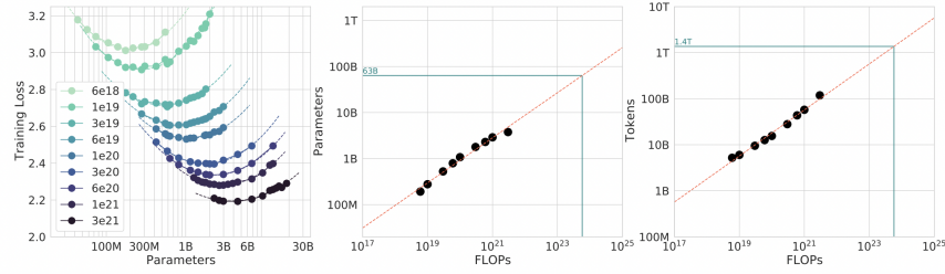
Рис. 84: Анализ IsoFLOPs
