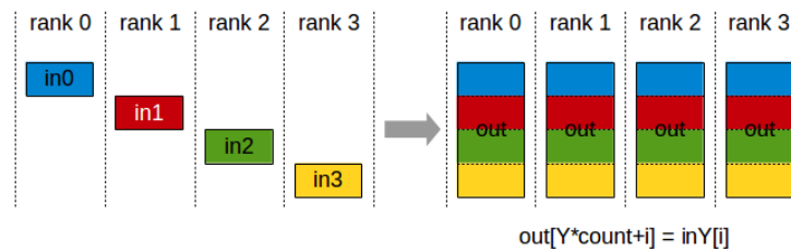
Рис. 39: Схема AllGather.
