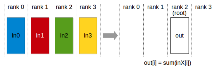
Рис. 40: Схема Reduce.
