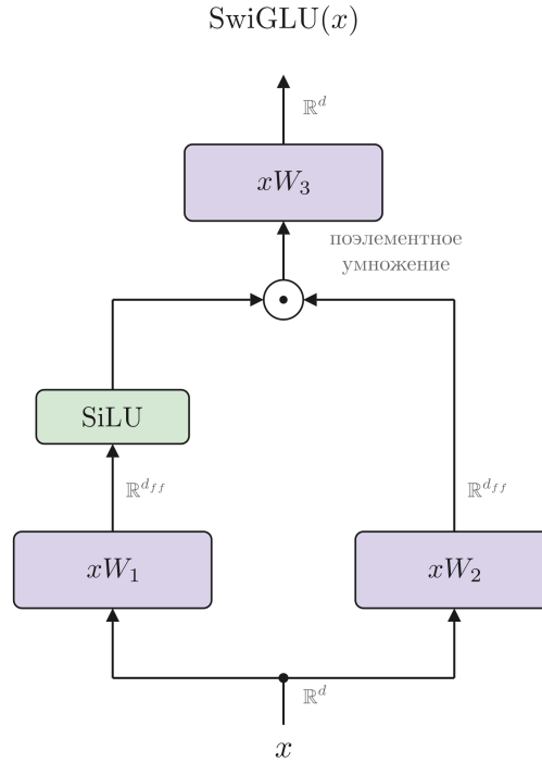
Рис. 65: Схема SwiGLU-блока.
