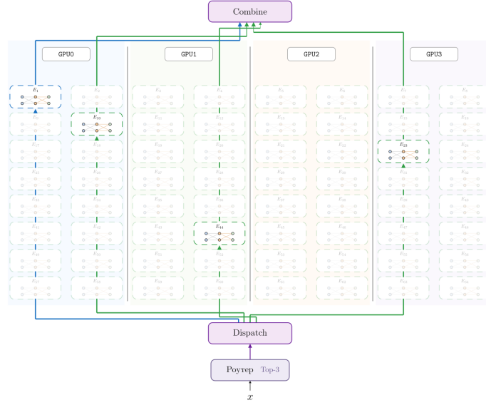
Рис. 90: Схема экспертного параллелизма (EP).
