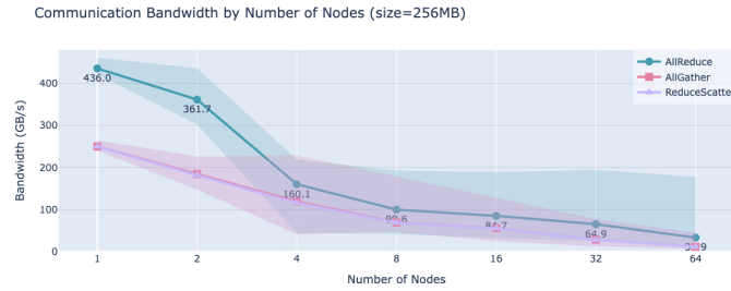
Рис. 60: Пропускная способность межнодовой коммуникации в зависимости от количества нод. Взято из Ultra-Scale Playbook.
