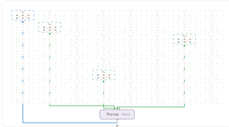
Рис. 89: Схема МоЕ-слоя с общими экспертами. Общие эксперты обрабатывают каждый токен.
