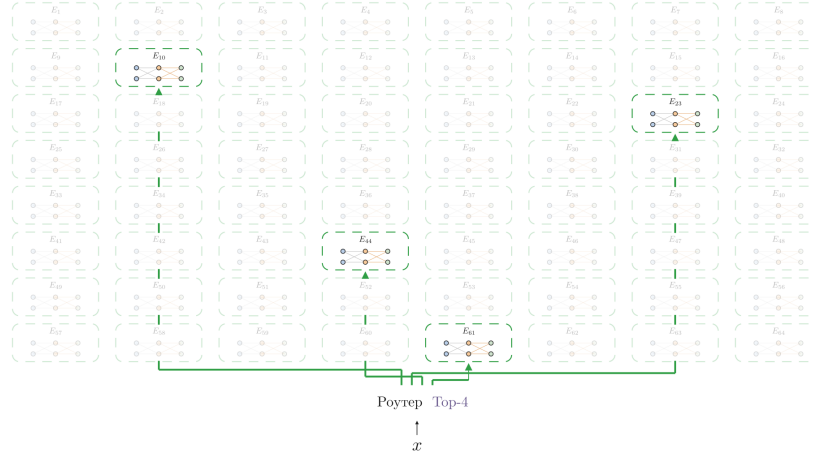
Рис. 88: Схема МоЕ-слоя с мелкозернистыми экспертами.
