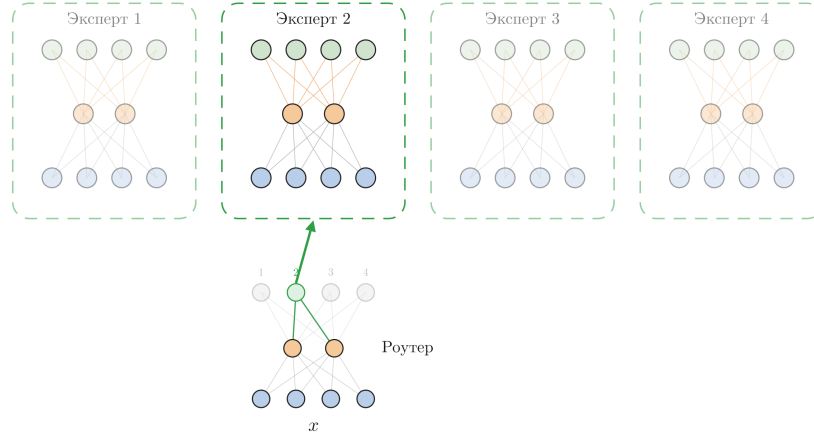
Рис. 87: Схема МоЕ-слоя. Маршрутизатор выбирает наиболее релевантные эксперты для каждого токена (в данном случае - только одного эксперта из четырех).
