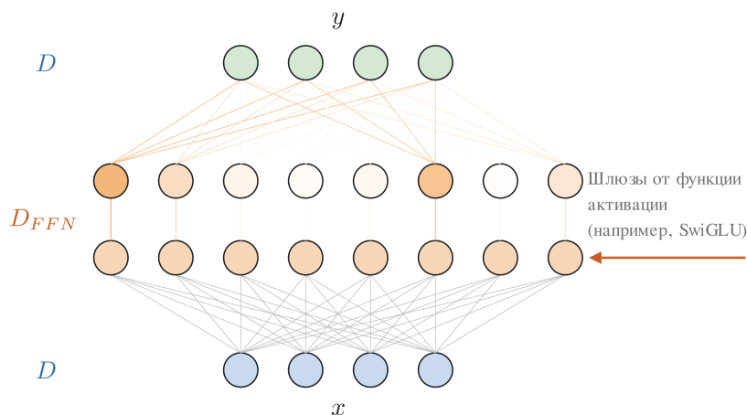
Рис. 85: Схема FFN-блока. Функция активации отсекает нерелевантные концепции, как бы "гася" их.
