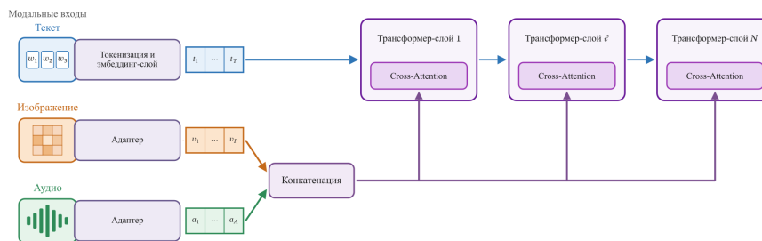
Рис. 78: Схема глубокого смешивания модальностей. Поскольку замешивание модальностей происходит на каждом слое, то и дообучение модели становится более дорогим
