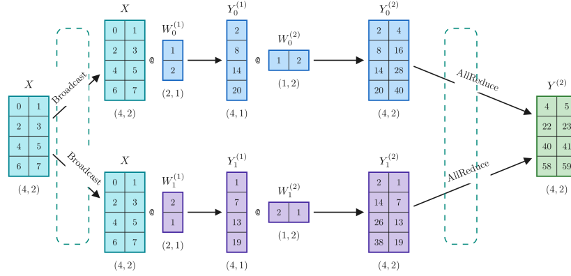
Рис. 54: Схема вычисления FFN-блока с использованием сначала параллелизма по столбцам, а следом — параллелизма по строкам.
