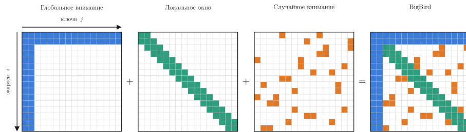
Рис. 71: Маска внимания в шаблонном разреженном внимании.
