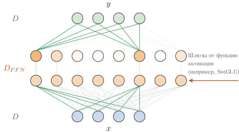
Рис. 86: Если токёну x соответствует лишь малая часть концепций, то зачем нам хранить и вычислять все остальные?
