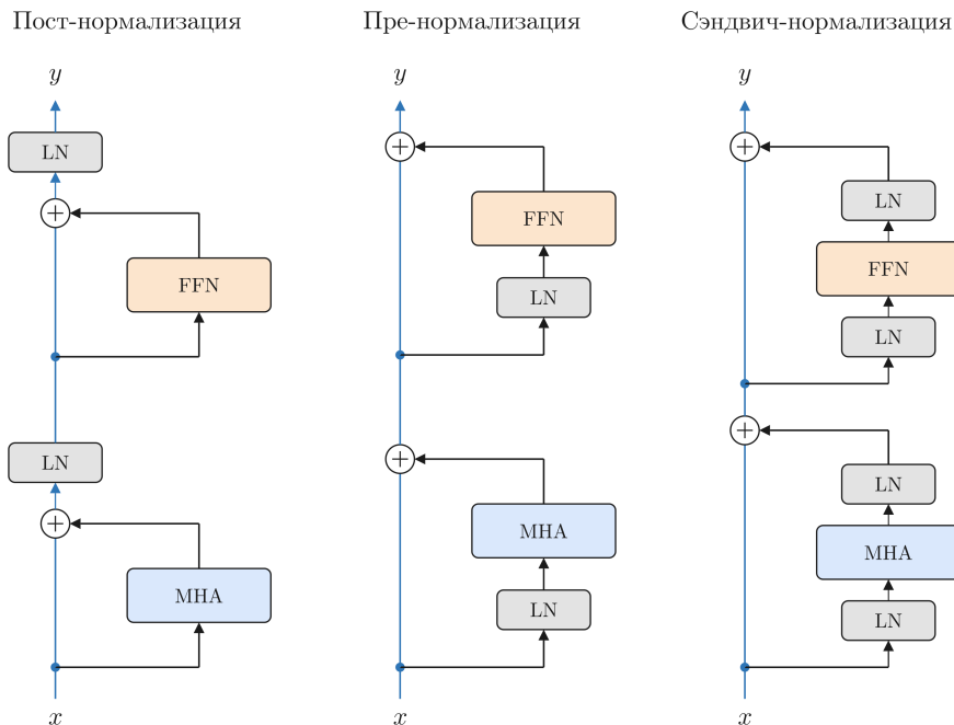
Рис. 64: Схемы пре-нормализации, пост-нормализации и сэндвич-нормализации.
