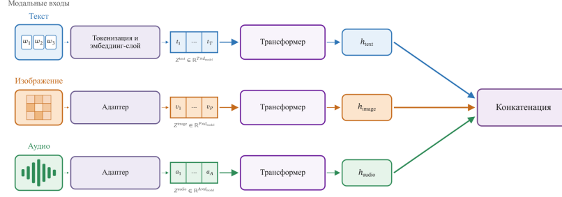
Рис. 79: Схема позднего смешивания модальностей.
