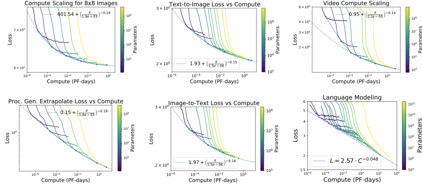
Рис. 82: Законы масштабирования для различных доменов
