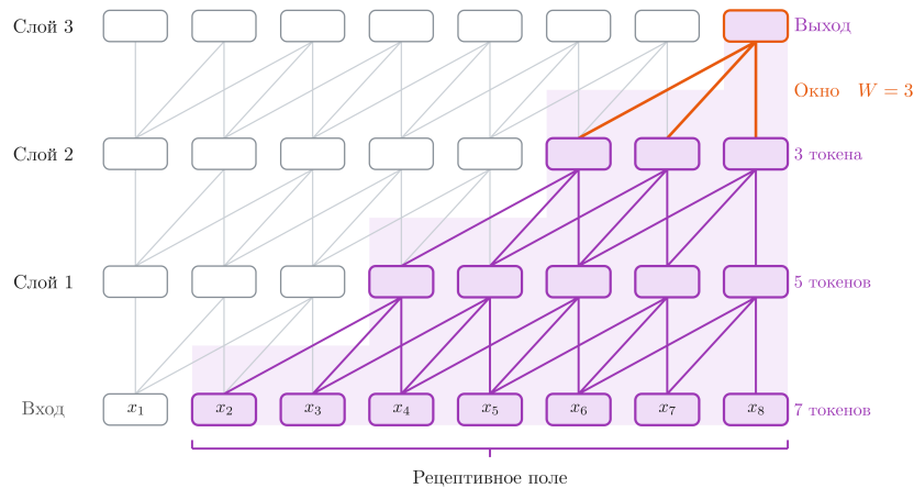
Рис. 73: Поле восприятия при скользящем оконном внимании.
