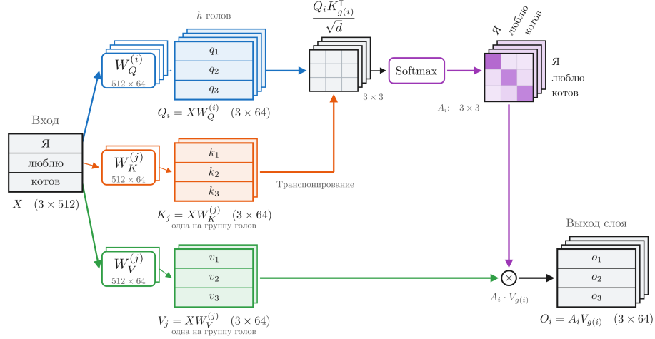
Рис. 69: Схема Grouped-Query Attention.
